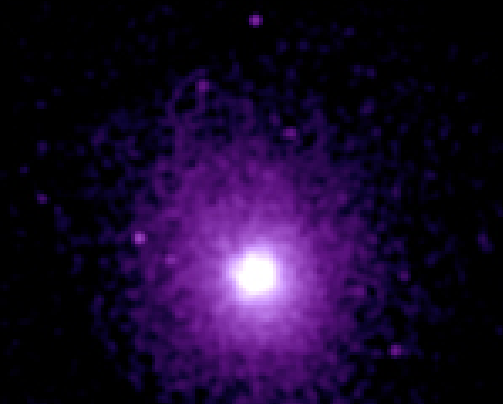
Abell 1689
