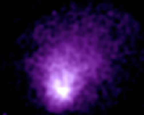
Abell 665
