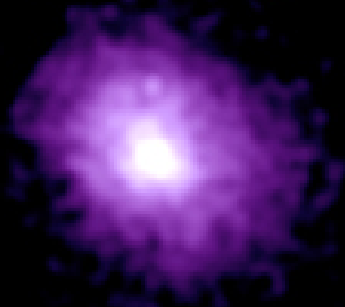
CL 0016+1609
