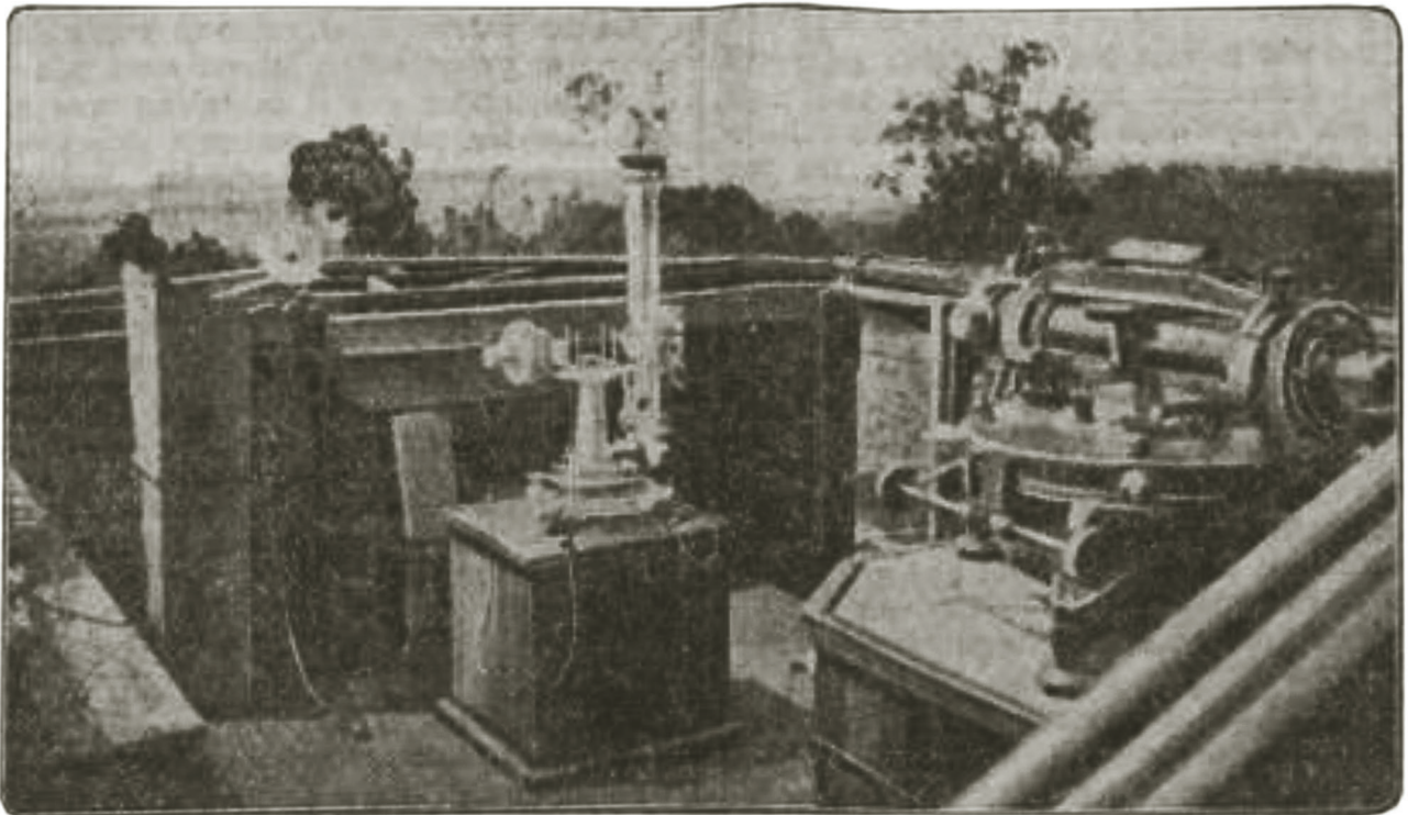
Rechts: het nieuwe model azimuth-instrument; midden: zenith-telescoop; links achtergrond: chronograaf met strokenbak; links: cellenkast, schakelbord en radioapparaten
