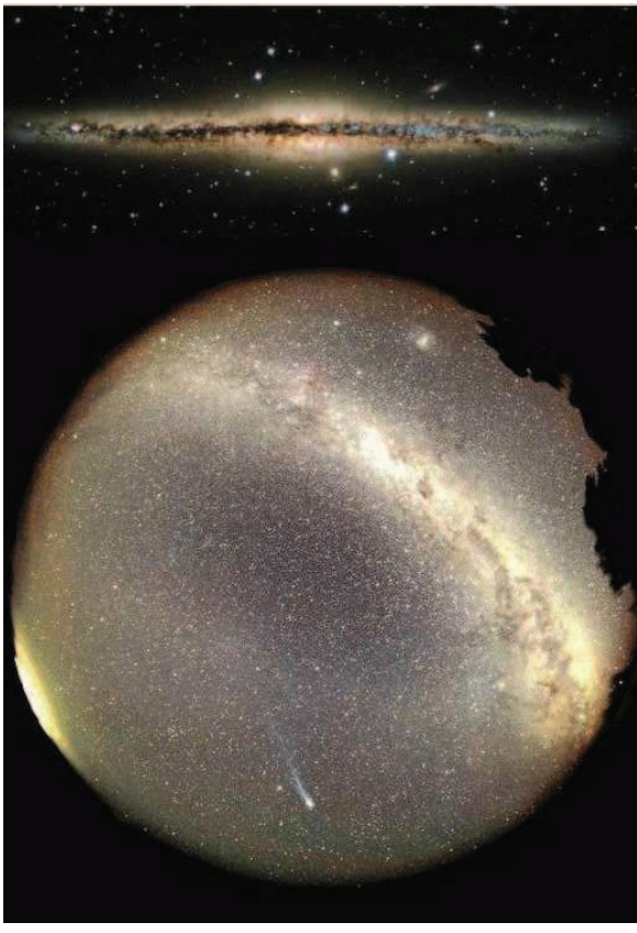
Figuur 26. Links een wijdhoekfoto van de gehele zuidelijke hemel. De rand van de opname is de horizon. We zien de Melkweg met rechts de Magelhaense Wolken, die begeleiderijes zijn van ons eigen Melkwegstelsel. Ook zien we op deze opname links de komeet Hyakutake. Deze foto is gemaakt in maart 1992 en was Astronomy Picture of the Day op 10 maart 2002. (antwpr.gsfc.nasa.gov/apod/ap020310.html; credit: Gordon Garradd (www.panoramio.com/photo/3233228)) Rechts het melkwegstelsel op z'n kant NGC 891, waar ik veel onderzoeken aan heb gedaan en ook heb benadrukt dat het heel veel op ons eigen stelsel lijkt. (www.cfit.hawaii.edu/HawaiianStarlight/English/Poster-NGC891.html; credit: The Canada-France-Hawaii Telescope CFHT, which is operated by the National Research Council of Canada, the Centre National de la Recherche Scientifique of France and the University of Hawaii.)
