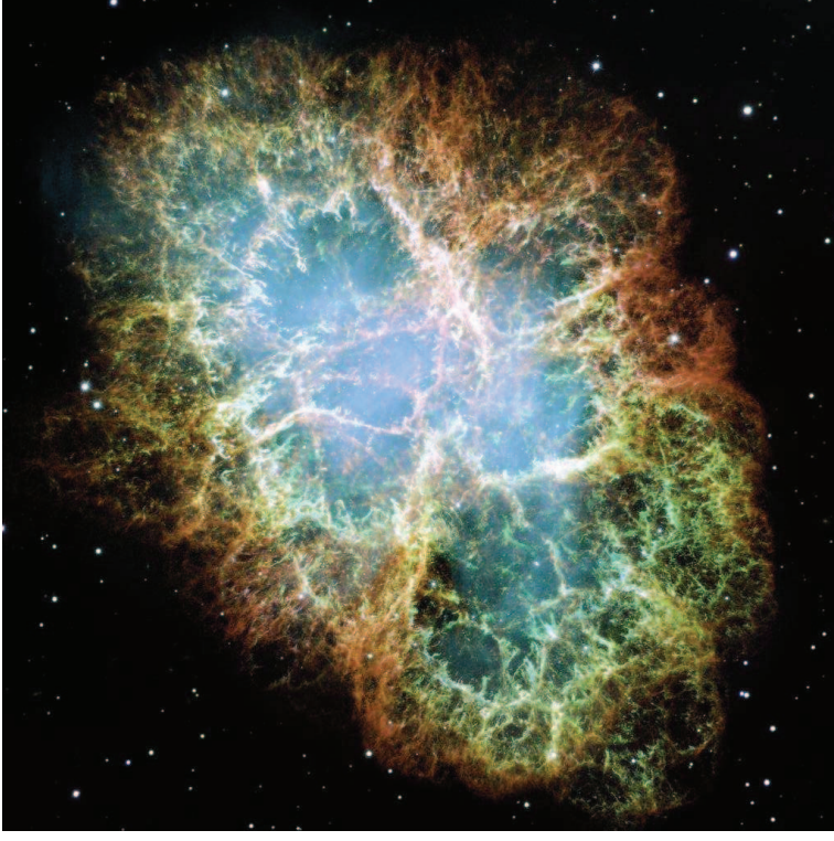
Figuur 34. Massieve sterren leven kort en blazen zichzelf op aan het eind van hun leven als een supernova, waarbij ze de chemische elementen die ze gevormd hebben aan het gas tussen de sterren toevoegen. Hier zien we de zogenaamde 'Krab-nevel', wederom met Hubble Space Telescope. Het is het restant van een supernova explosie die op aarde in 1054 met het blote oog zichtbaar was. (hubblestte.org/gallery/album/nebula_collection/pr2005037a/; credit: STScI.)
