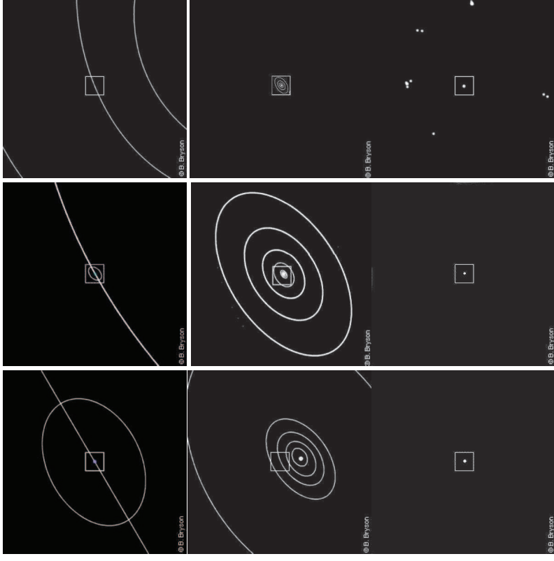
Figuur 16. De machten van tien volgens Bryson (2005) van de schaal van een miljoen kilometer ( 10^6 meter) tot die van 100 miljard kilometer ( 10^{17} meter). Het is beter dit uit te drukken in lichtjaren en de laatste schaal is dan ongeveer 10 lichtjaar. Ik heb uit de plaatjes van het zonnestelsel de baan van Pluto verwijderd. (credit: see fig. 12)
