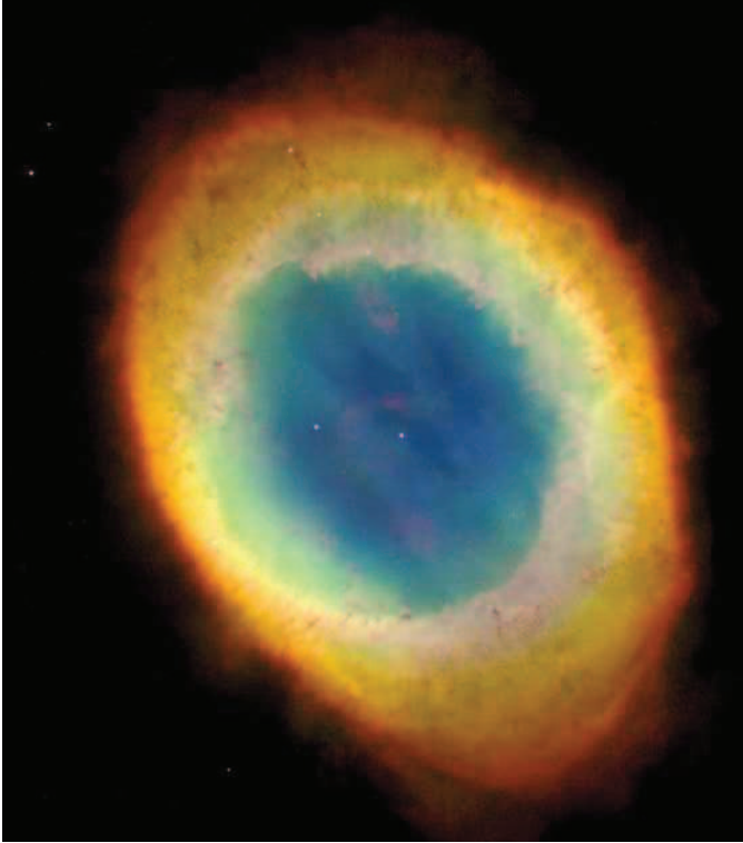
Figuur 32. De 'Ringnevel', een voorbeeld van een planetaire nevel, op een opname met de Hubble Space Telescope. Dit object staat op een afstand van ongeveer 2300 lichtjaar. (heritage.stsci.edu/1999/01/images/9901a.jpg; credit: STScI.)
