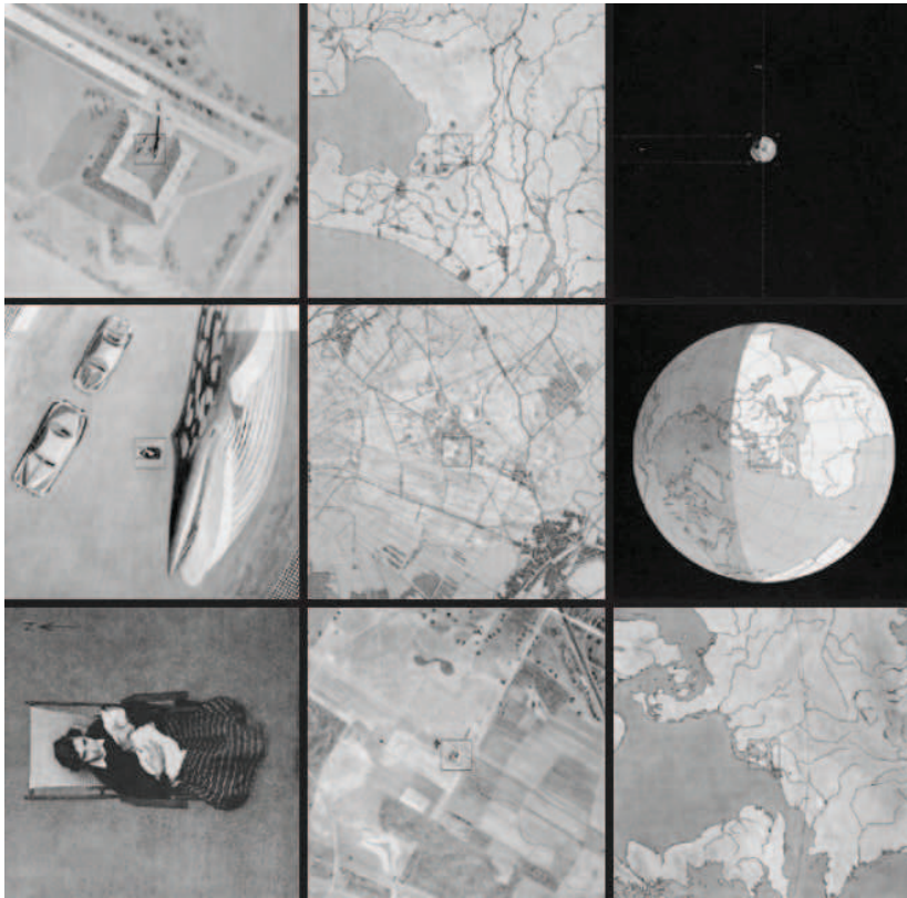
Figuur 11. De negen eerste plaatjes van Kees Boeke. Linksboven meet 1,5 bij 1,5 meter en de volgende worden telkens een factor tien groter, zodat rechtsonder 150,000 bij 150,000 kilometer beslaat. (credit: nedw-ww.ipac.caltech.edu/level5/Boeke/frames.html)
