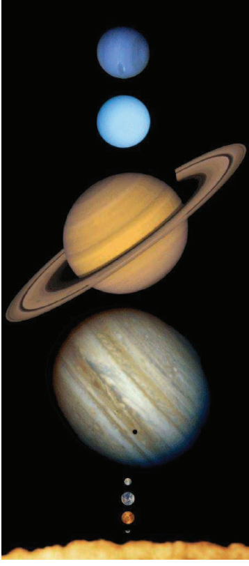
Figuur 36. De planeten van ons zonnestelsel op dezelfde schaal in afmeting, maar niet in afstand tot de zon. Ze staan wel op de goede volgorde, namelijk van binnen naar buiten Mercurius, Venus, aarde, Mars, Jupiter, Saturnus, Uranus (klein toon op de eerste lettergreep) en Neptunus. Ik heb Pluto uit deze foto verwijderd. (see: jpl.nasa.gov/multimedia/gallery/solarsys.scale.jpg ; credit: The Jet Propulsion Laboratory JPL of the National Aeronautics and Space Administration NASA at the California Institute of Technology Caltech.)
