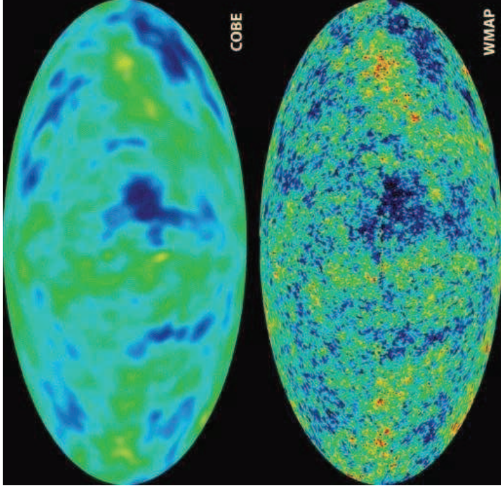
Figuur 21. Dit is een kaart van de fluctuaties in de helderheid van de kosmologische achtergrondstraling. We zien de hele hemel opengeklapt net als een kaart van de hele aarde. De fluctuaties zijn op het niveau van ongeveer 0.01% en tonen de eerste structuur in het heelal. Het bovenste plaatje is begin jaren negentig gemaakt met de satelliet Cosmic Background Explorer COBE, wat de Nobelprijs heeft opgeleverd. Onder een meer recente bepaling met de Wilkinson Microwave Anisotropy Probe WMAP. (credit: The National Aeronautics and Space Administration (NASA) and the WMAP Science Team; zie map.gsfc.nasa.gov/media/080997/index.html )
