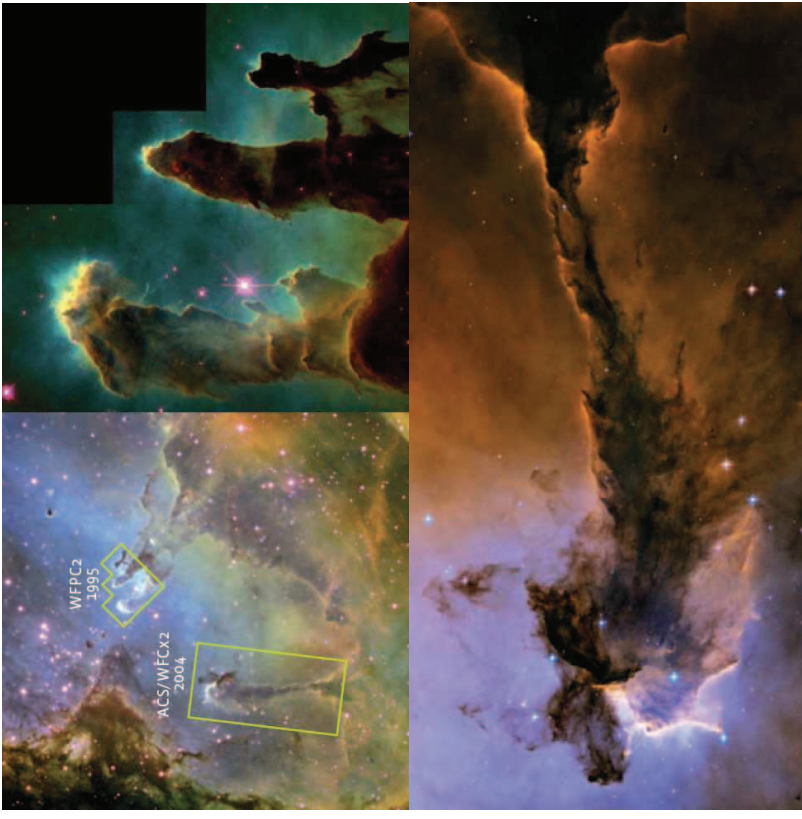
Figuur 29. Vorming van sterren in de zogenaamde Arend-nevel. Deze nevel (linksboven) is een kraamkamer van sterren, die in grote getale op dit moment vormen. Onder de jonge sterren zijn er, die veel zwaarder zijn dan de zon en zulke jonge sterren zenden veel ultraviolet licht uit, waardoor het gas gaat gloeien. We zien het dan afsteken tegen het stof in deze opnamen rechtsboven en onder met Hubble Space Telescope. De nevel ligt 6500 lichtjaar bij ons vandaan. ( heritage.stsci.edu/2005/12b/supplemental.html ; credit STScI.)
